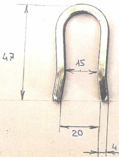
СКОБА \varnothing 12 мм (Р-12)
